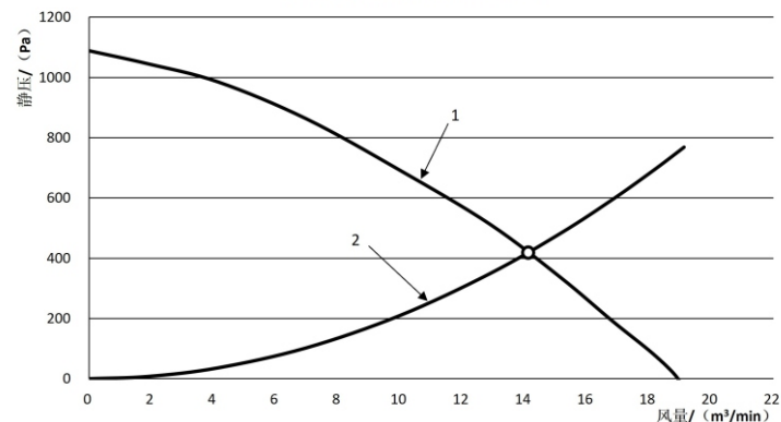
空气性能特性曲线及阻力曲线
