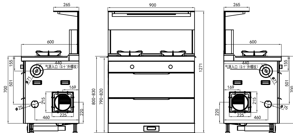
图二、产品尺寸示意图 单位 mm
