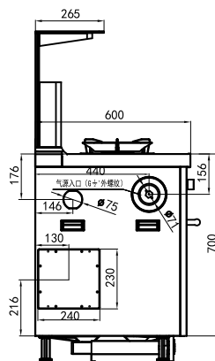
左出风
