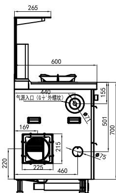
左出风
