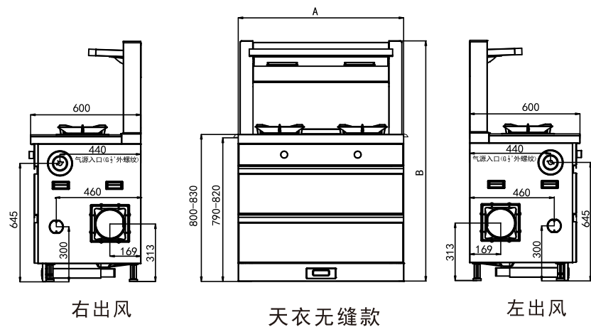
产品尺寸列表
