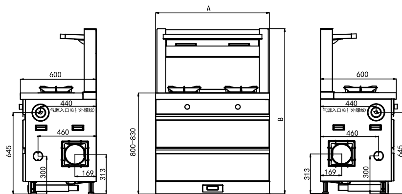
图二、产品尺寸示意图 单位 mm
