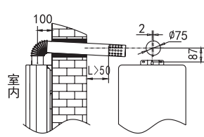
烟管背向安装 (图4)
